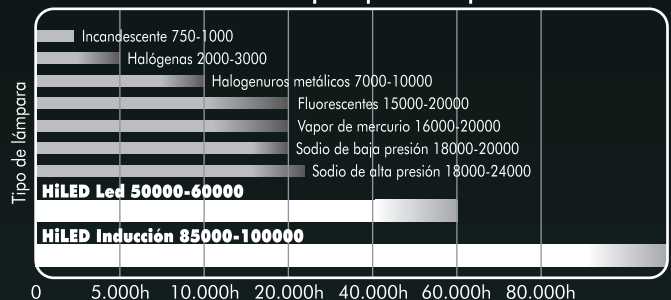
Vida media por tipo de lámpara
